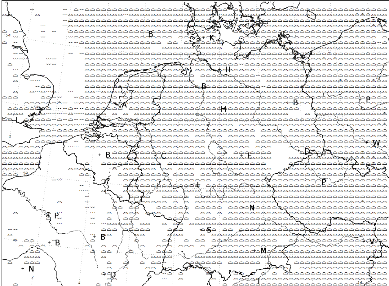
Identifier of humidity convection VT: 06 UTC Wed 17 Jul [ICON6_NEST 2019-07-15 12 UTC +42h] © 2019 Deutscher Wetterdienst
